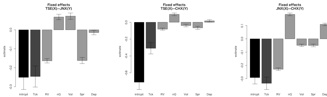
図5 回帰係数推定値および95%信頼区間-1: 左から、 y -切片、ティックサイズ変更効果 ( Tck )、実現ボラティリティ比 ( RV )、気配更新件数比 ( nQ )、約定枚数比 ( Vol )、スプレッド対仲値比 ( Spr )、デプス ( Dep ) の各変数。ティックサイズ変更効果は変更前後の変化量。5つの説明変数の係数推定値はティックサイズ変更前の値。東証(TSE)-JNX(左図)、東証-ChiX(中央図)、JNX-ChiX(右図)。 y 軸のプラス方向は、(他の変数が固定されている状態において)その説明変数の市場 Y の値が X よりも相対的に増加すると、市場 X の Y に対する先行度合が増加することを示す。
