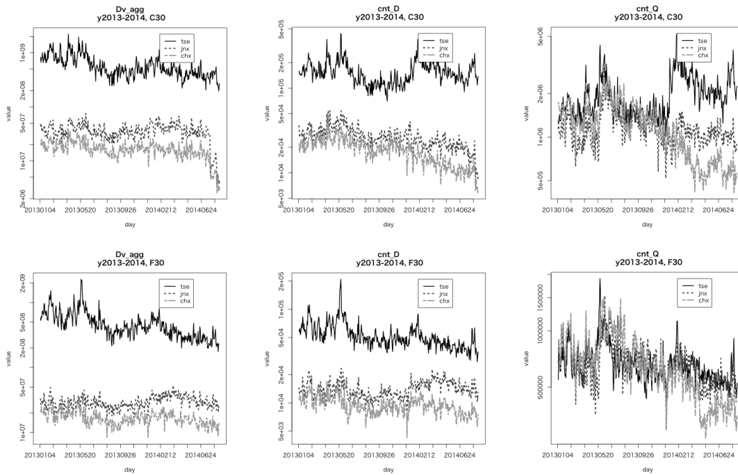
図1 日次時系列プロット-1: 出来高(約定枚数)の30銘柄合計値(左図), 約定件数の30銘柄合計値(中央図), 気配更新件数の30銘柄合計値(右図). Core30(上半分), FIX30(下半分). 各图中, 東証(TSE)は黒実線, JNXは濃い灰色点線, ChXは灰色鎖線で表示.
