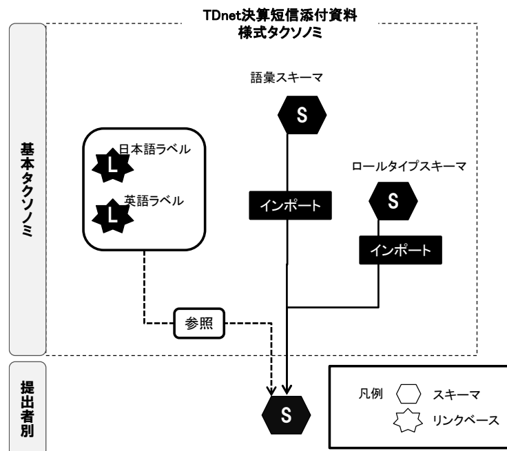
図 2 TDnet 決算短信添付資料様式タクソノミの参照・インポート
